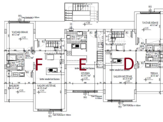
I. KAT PLANI
